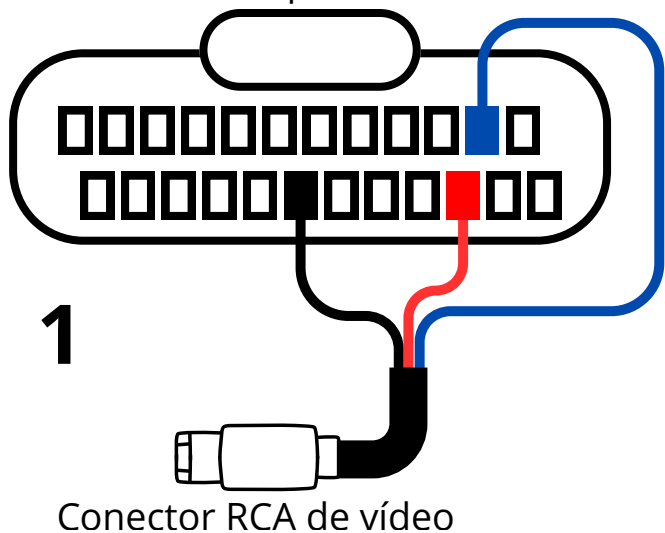
Conector visto pelo lado dos fios
