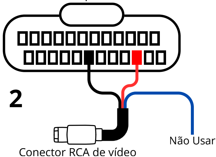
Conector visto pelo lado dos fios
